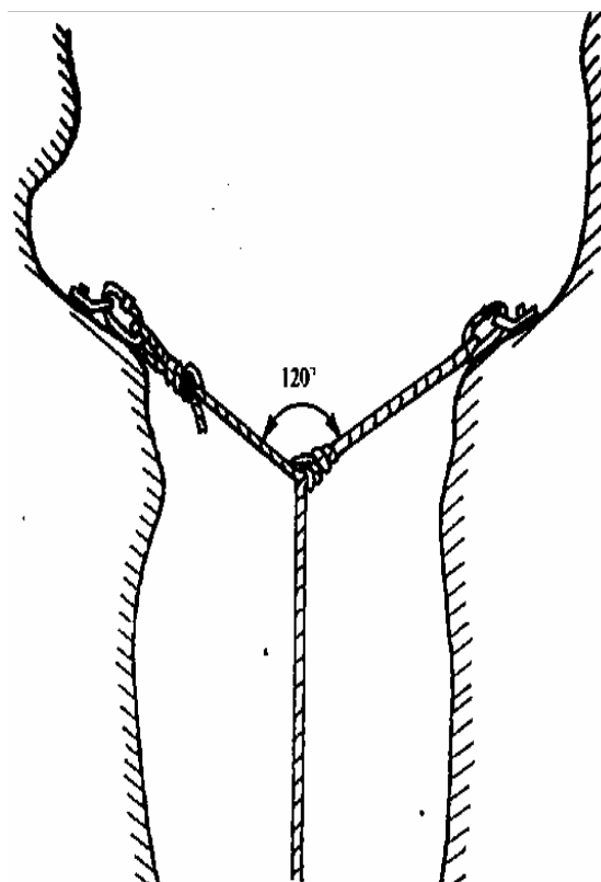
Фиг 26 Закрепване "У" между стени с раздвижен профил
