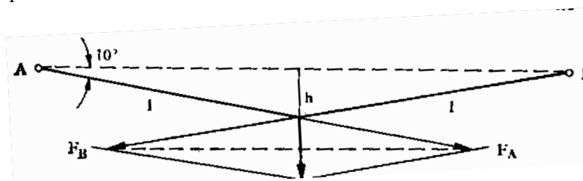
Фиг. 21. Схема за силите при натоварване на хоризонтално опънато въже
