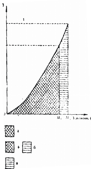
Фиг.6 Сигурност на въжето 1-практическа якост на опън; 2-ВДН при поемане на удара; а-енергия на падане, погълната от въжето; б-енергия, необходима за скъсване на въжето, с възли, мокро, замърсено и пр.; в-зона, в която се простира сигурността на вужето. Колкото стойността на ВДН2 се доближава до стойността на практическата якост на опън(1) толковаповече тази зона се стеснява, като намалява сигурността на въжето , и обратно.
