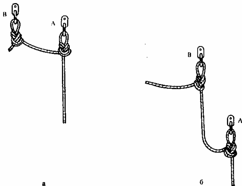
Фиг. 13. Оптимални разстояния между дублирани закрепвания: а — хоризонтално; б — вертикално дублиране
