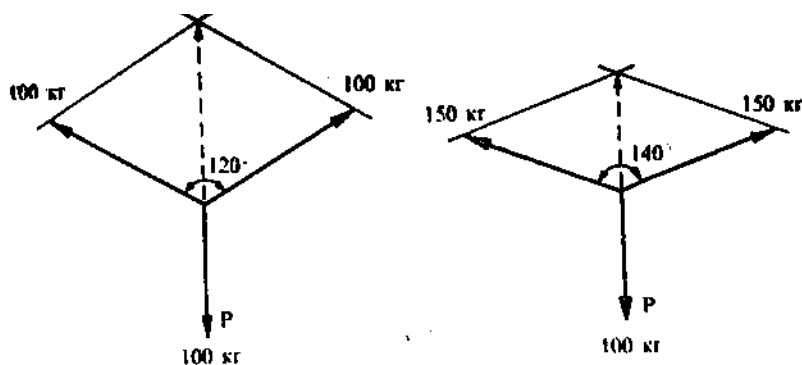
Фиг. 22. Натоварване на закрепване “У” при различни ъгли между рамената
