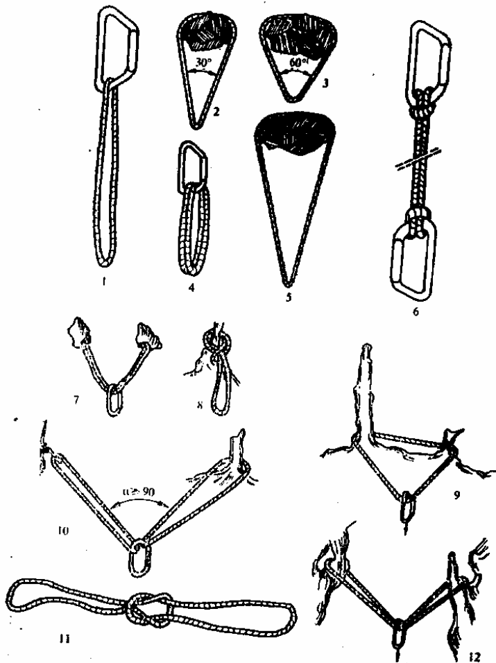
Фиг. 43. Въжени примки: 1 – единична, 4 – сдвоена, 6,8,9,12 – неправилно използване 1,2,3,4,5,7,10 – правилно използване 11 – съединяване на примки
