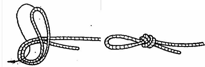
Фиг.38 Водачески възел
