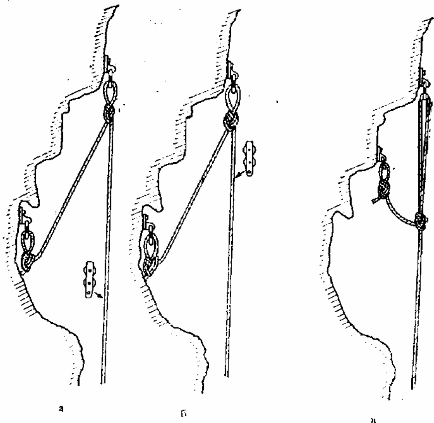
Фиг. 14. Оборудване на основно закрепване, разположено над допълнителното: а, б — неправилно; в — правилно
