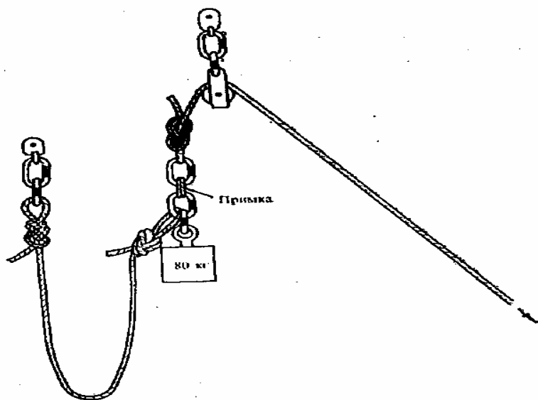
Фиг. 50. Установка за проверка на годността на статични въжета
