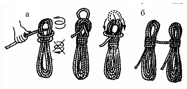
Фиг. 48. Навиване на въжета: а — единичен пакет; б — двоен пакет
