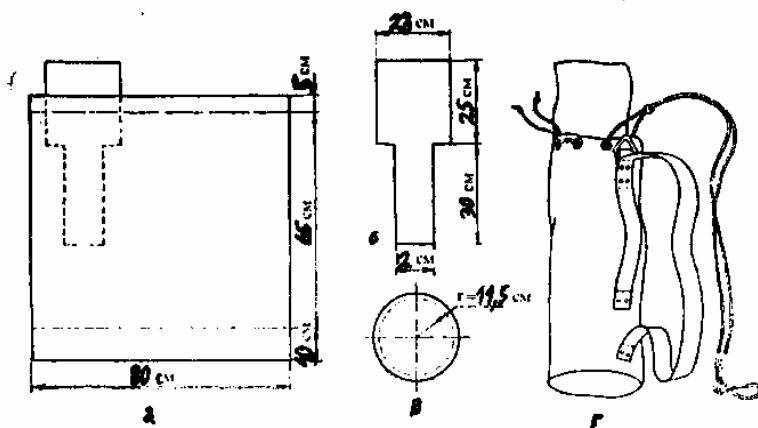
Фиг. 49. Транспортен сак:
