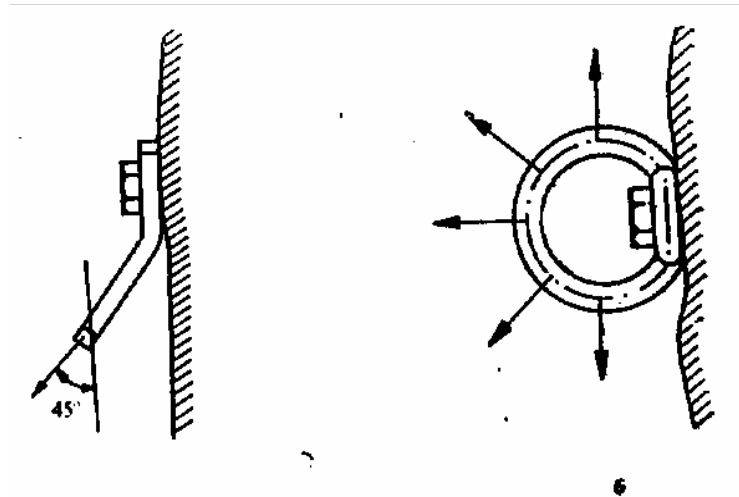
Фиг.24 а-профилна планка; б- таванна планка
