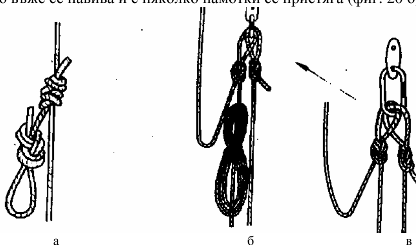
Фиг. 20. Свързване на две въжета: а — камбана; б, в — към междинно закрепване
