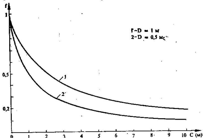
Фиг. 29. Зависимост на фактора на падане от дължината на въжето С над междинното закрепване и големината на «корема» D
