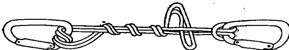
Фиг. 41. Възел «Маринер»
