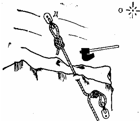
Фиг. 15. Неправилно дублирано основно закрепване: О — основно закрепване; Д — допълнително закрепване
