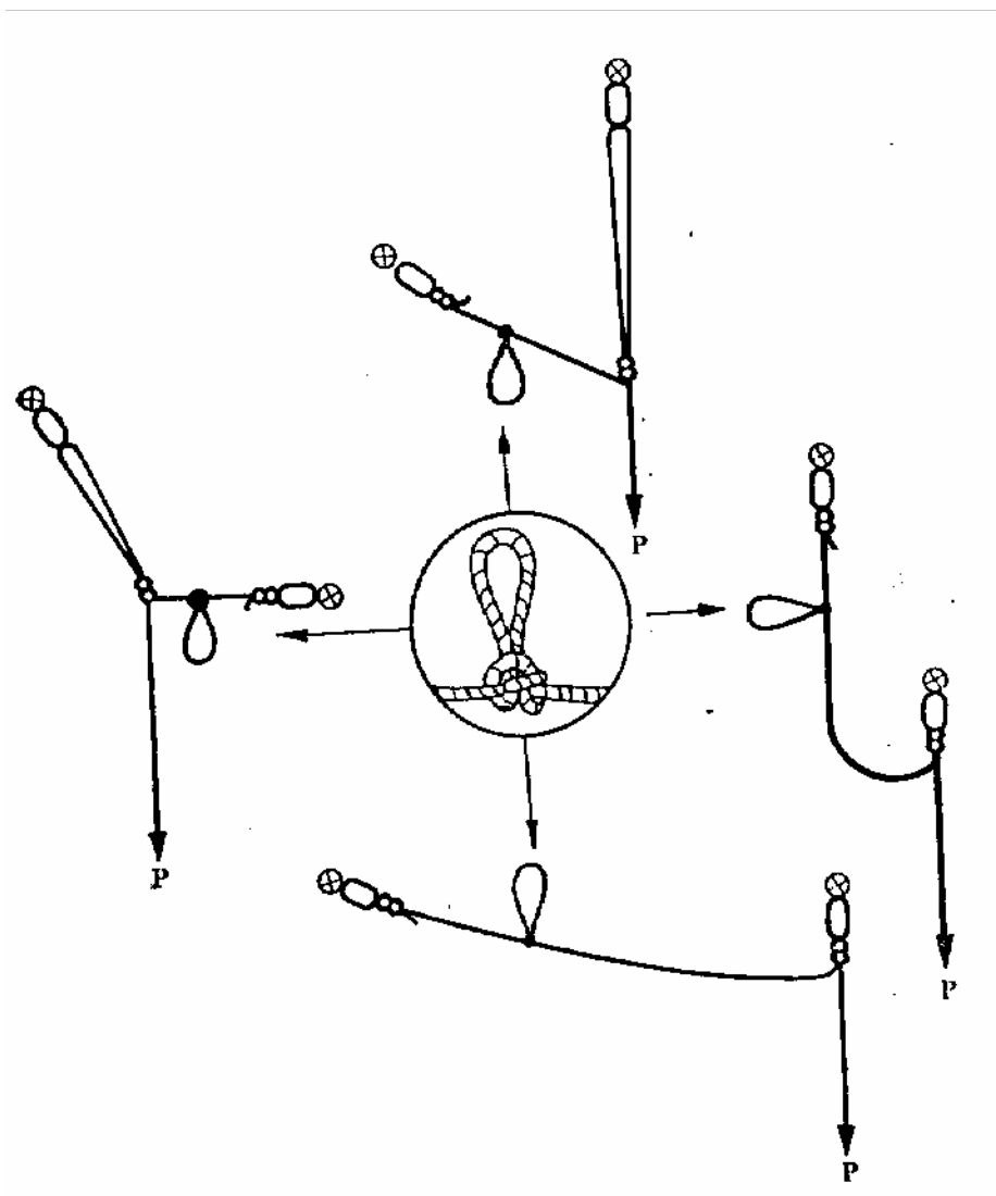
Фиг. 16 Амортизиращ възел и схема на закрепванията, при които се използва
