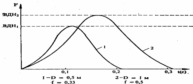
Фиг 31. Теоретични криви на ВДН при еднакви значения за S и F , но различна големина на «корема» D
