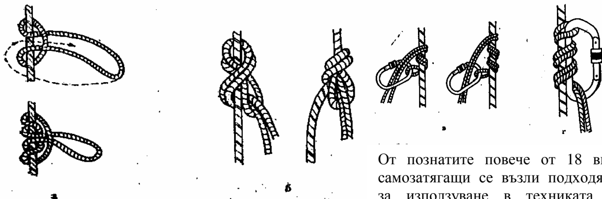
Фиг 37 а – “Прусик”; б-кръстосан; в – арб; г – “Бахман”
