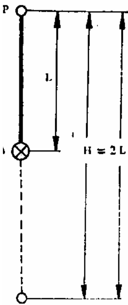
Фиг. 4. Фактор па падане: а — при H=2L , f=2 ; б — при H=L , f=1
