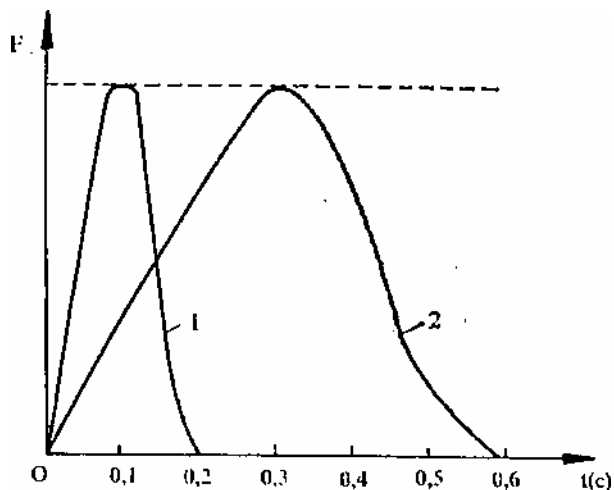
Фиг. 5 Продължителност на импулса на силата.
