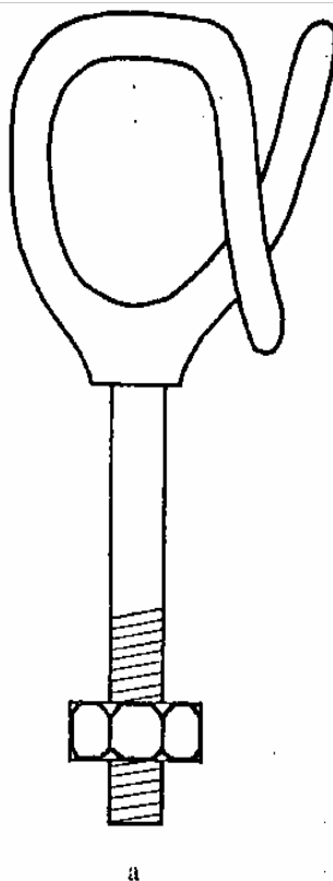
Фиг.18 Отклонител а-общ вид; б-начин за използване
