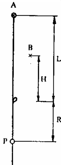
Фиг.28 Фактор на падане при разрушаване на междинно закрепване
