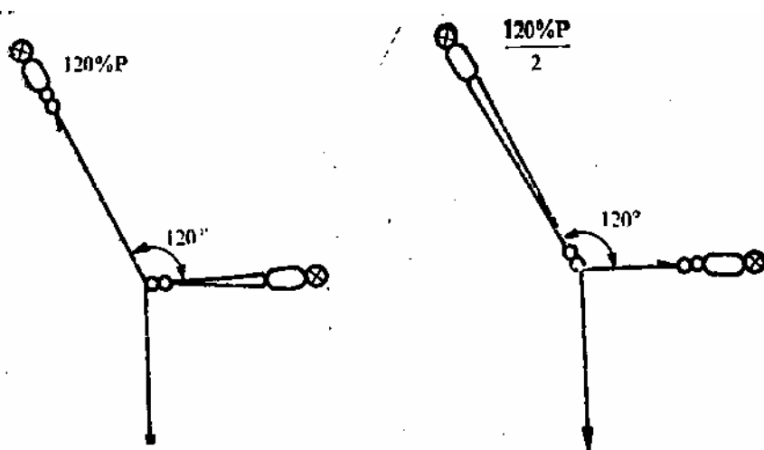
Фиг. 23 Намаление на натоварването чрез вдвояване на въжето, фиксирано към по-висока опора на закрепването.
